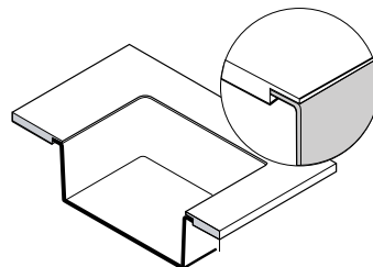
Semi-underlimmad / Underfräst
